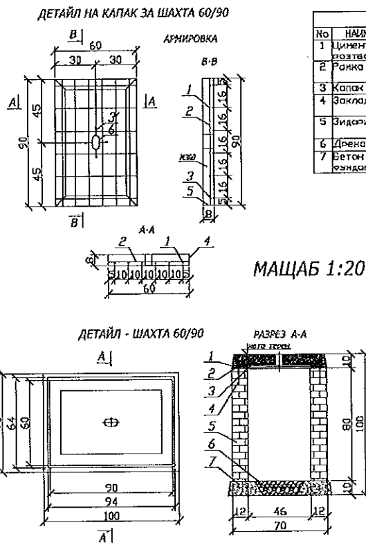
Фиг. 6.3. Кабелна шахта – единична
